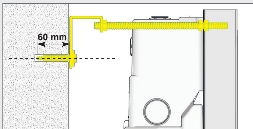
vue de profil - zijanzicht - Side view
