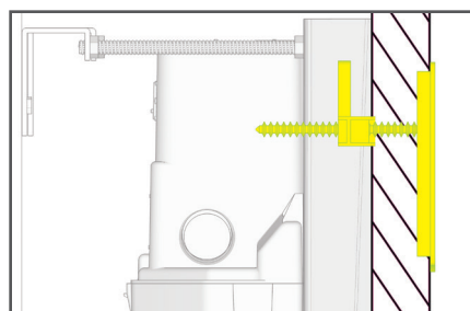
vue de profil - zij aanzicht - Side view
