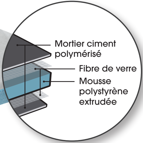
NATTE ÉTANCHE PRÉ-MONTÉE avec débord de 10 cm redécoupable
