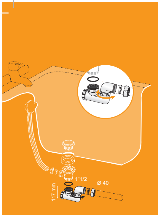
SIPHON DE BAÏGNOÏRE SIFON VOOR BAD
