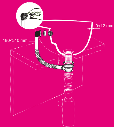
Lavabo avec trop-plein extérieur Wastafels met een externe overloop
