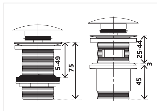
Clapet rotatif
