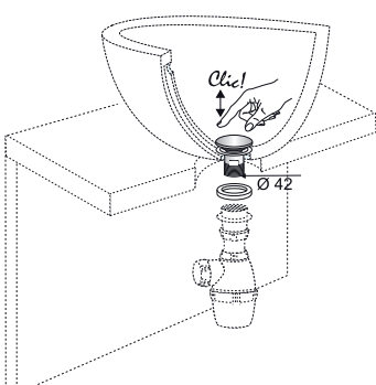
Lavabo avec trop-plein intégré Washbasin with integrated overflow
