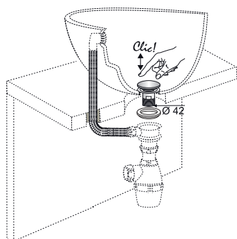
Lavabo avec trop-plein extérieur Washbasin with external overflow
